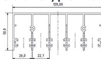
5-drážkový profil horní
