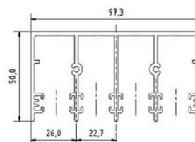
4-drážkový profil horní
