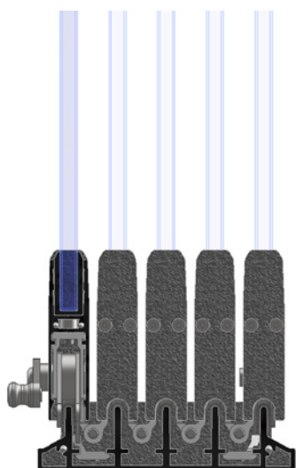
Řez spodní 5 kolejnice a pojezdového profilu
