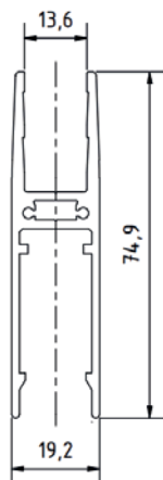
Pojezdový profil panelů
