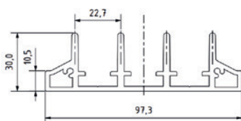
spodní 4-kolejnice
