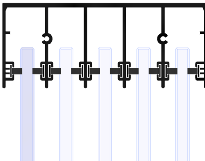
Horní 5 drážkový profil
