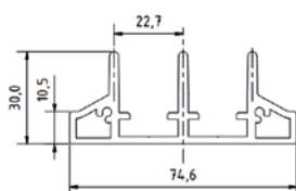
spodní 3-kolejnice
