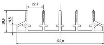
spodní 5-kolejnice
