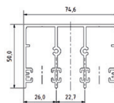
4-drážkový profil horní
