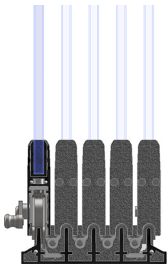
Řez spodní 5 kolejniče a pojezdového profilu
