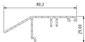
SKE-01 Krajní zasklívací lišta
