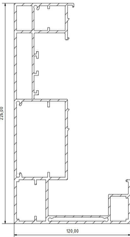
SKY-01 Obvodový profil
