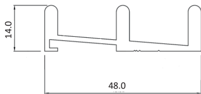
SLIDE-01 Vodicí profil spodní
