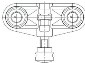
SLIDE-08-B Pojezd horní - Vozík
