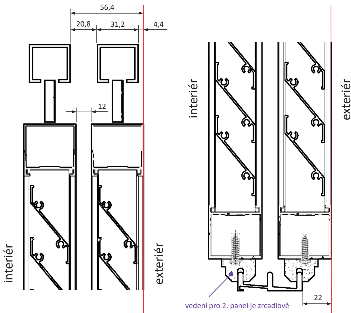
2 panely na 2 horních kolejničích – vedle sebe (2x posuvný slunolam vedle sebe)
