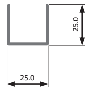
PRO200-11 U Profil 25x25
